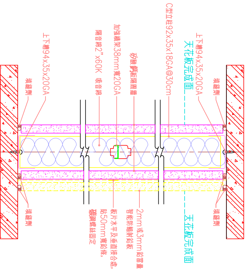
防輻射封板到頂—小時防火時效輕鋼架隔間牆 (2mm或3mm鉛當量智能防輻射鉛板)
